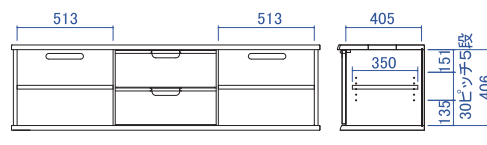
TVボード165H
