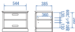
ローボードN65
