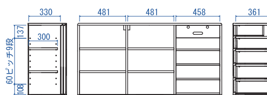
サイドボード150
