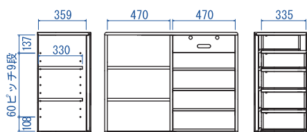
サイドボード100
