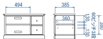
ローボードN85
